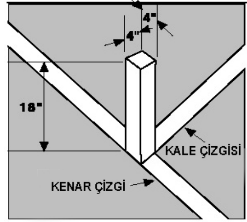
PİLON DETAYI
